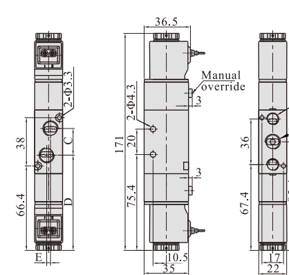
4V220(Grommet)
