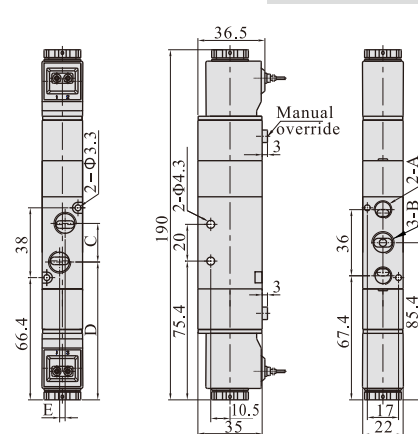
4V230(Grommet)
